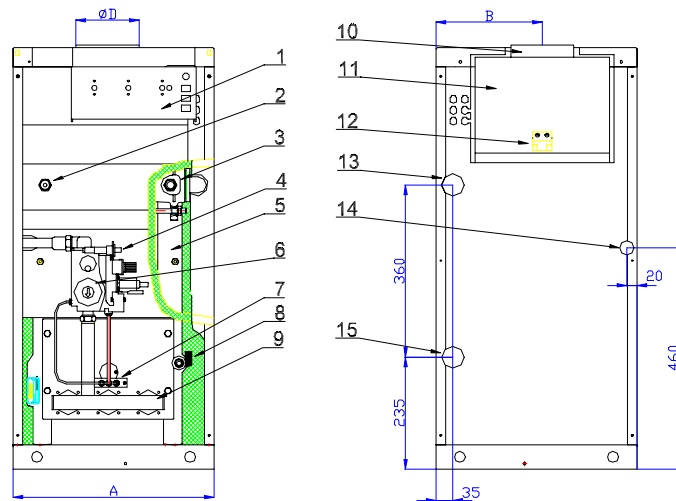
Рис.1 - Присоединительные и основные размеры котла
