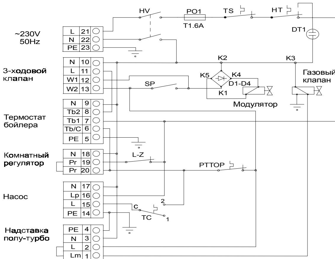
Рис. 4 – Схема электрического подключения котла 20, 30, 40, 50 PLO
