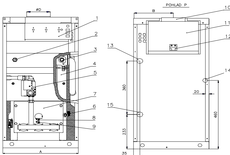
Рис. 1- Соединительные и основные размеры котла
