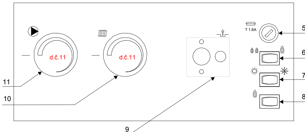
Рис.36 Панель управления вертикальная
