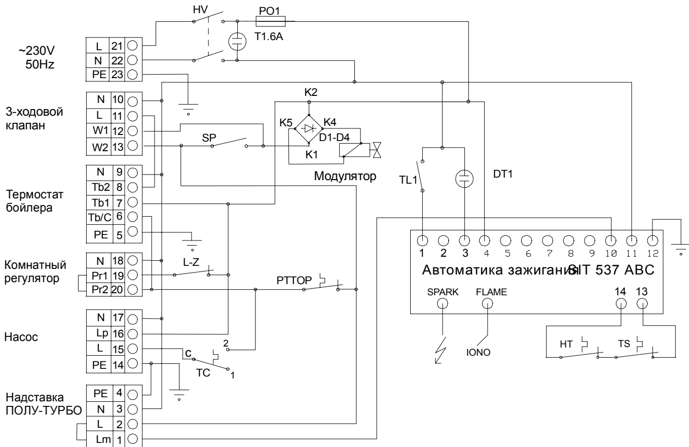
Рис. 46 – Схема электрического подключения 40, 50 KLO
