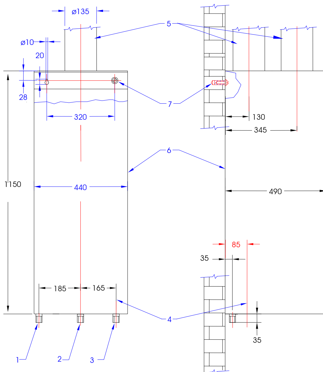
Рис. 2 Присоединительные размеры котла
